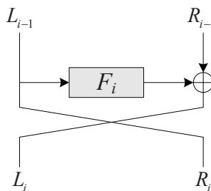
Fig. 1. Feistel Structure
