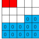
Fig. 4. Keccak-MAC-384
