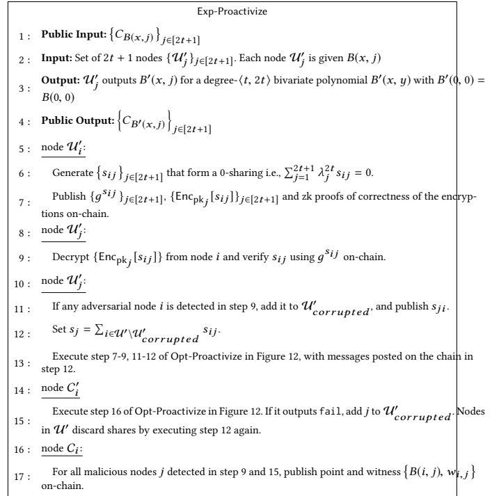
Fig. 16. Exp-Proactivize protocol.
