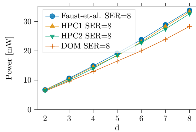
(b) SER = 8
