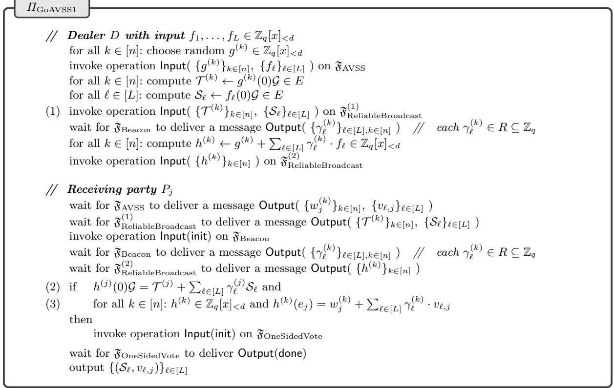
Fig. 6. A GoAVSS protocol
